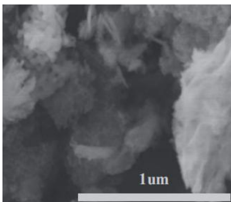
纳米氧化镁的 SEM 图 (1μm)
