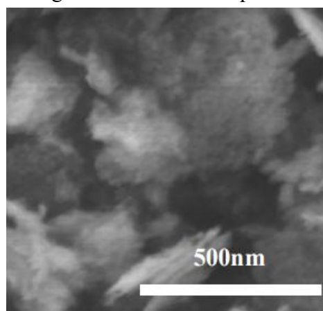
纳米氧化镁的 SEM 图 (500nm)
