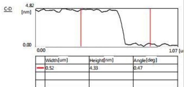
小片径薄层二硫化钨分散液的 AFM AFM image of Thin Layer Nano WS2 Dispersion
