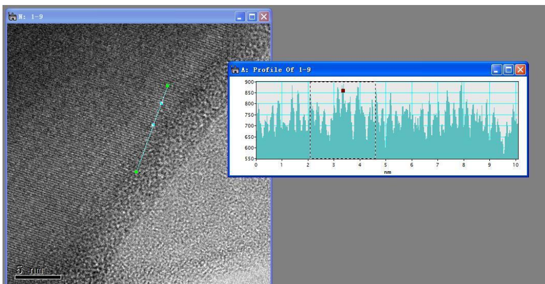
黑磷晶体的 HRTEM 图 HRTEM image of black phosphorus crystal
