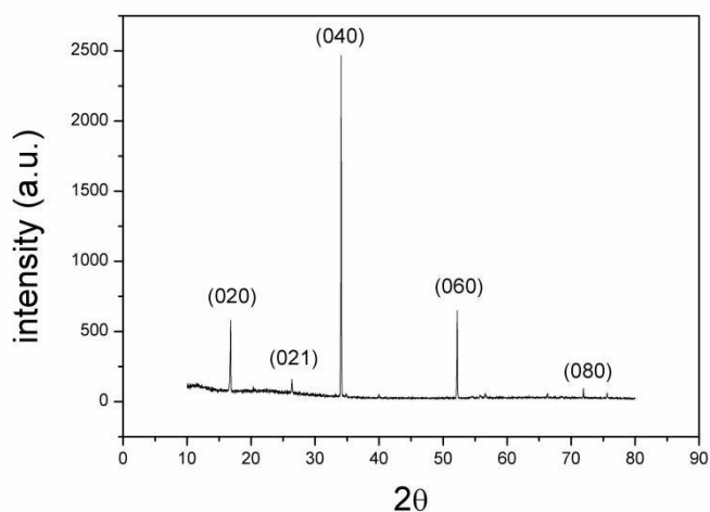
黑磷晶体的 XRD 图谱 XRD pattern of black phosphorus crystal
